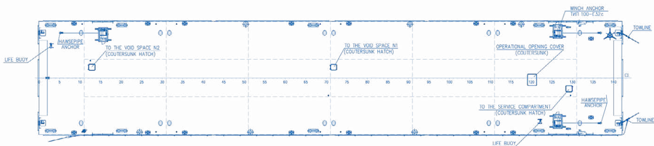
Вид сверху
