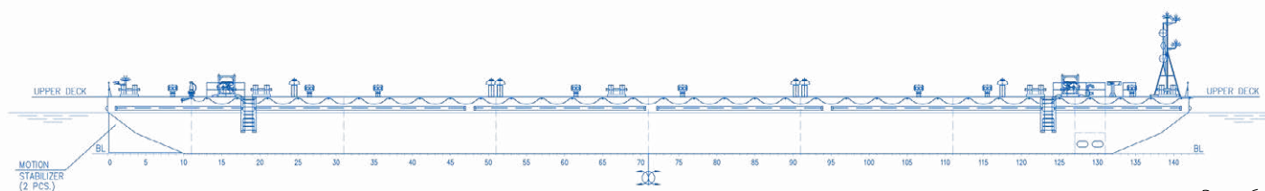
Вид сбоку
